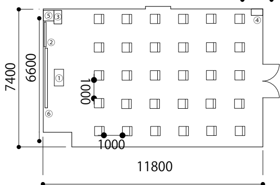
会議室5 W11800/D7400/H3000 シアター 30 席
